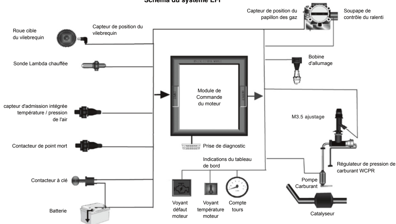
Schéma du système EFI
